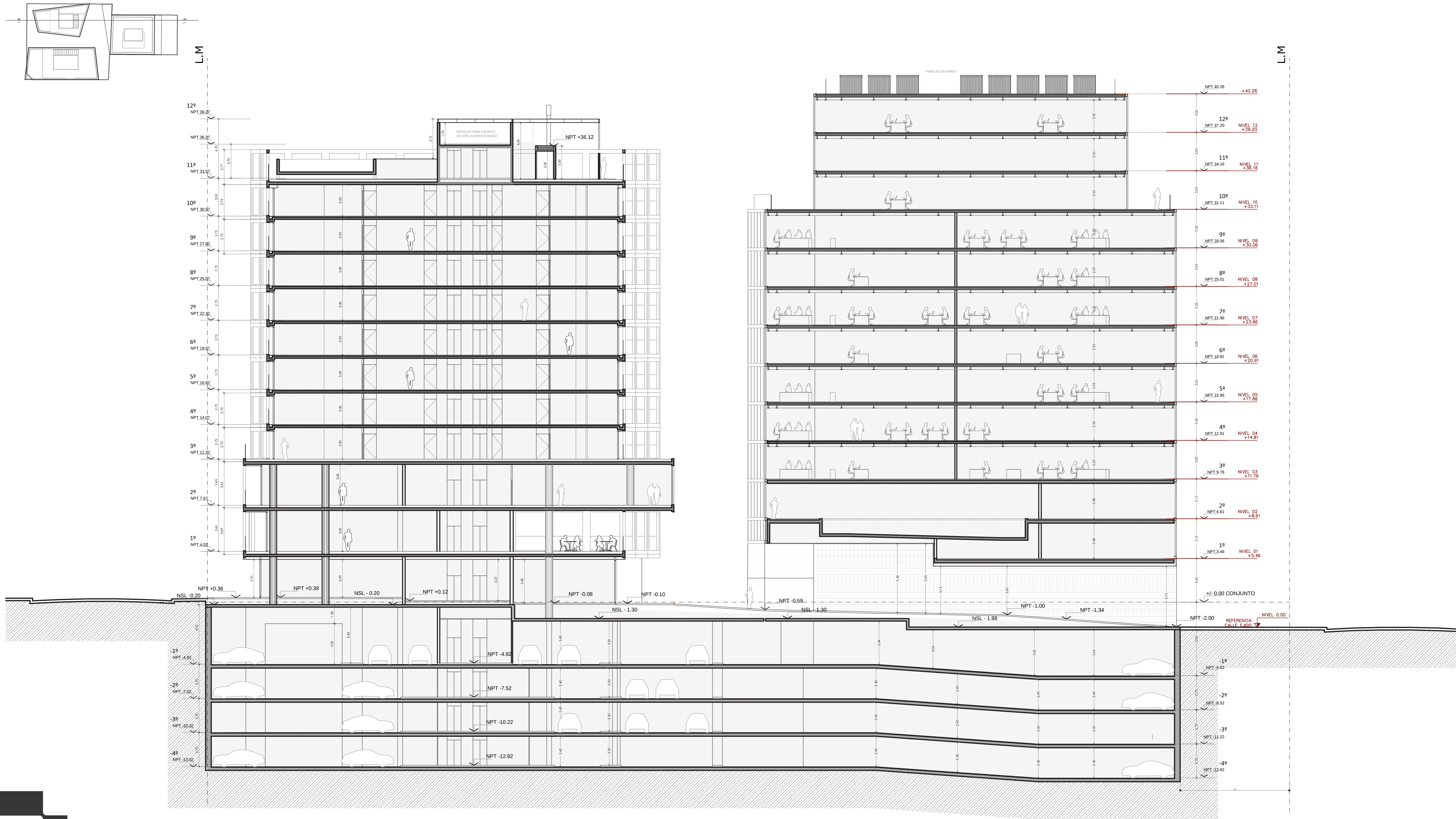
Corte Longitudinal A
