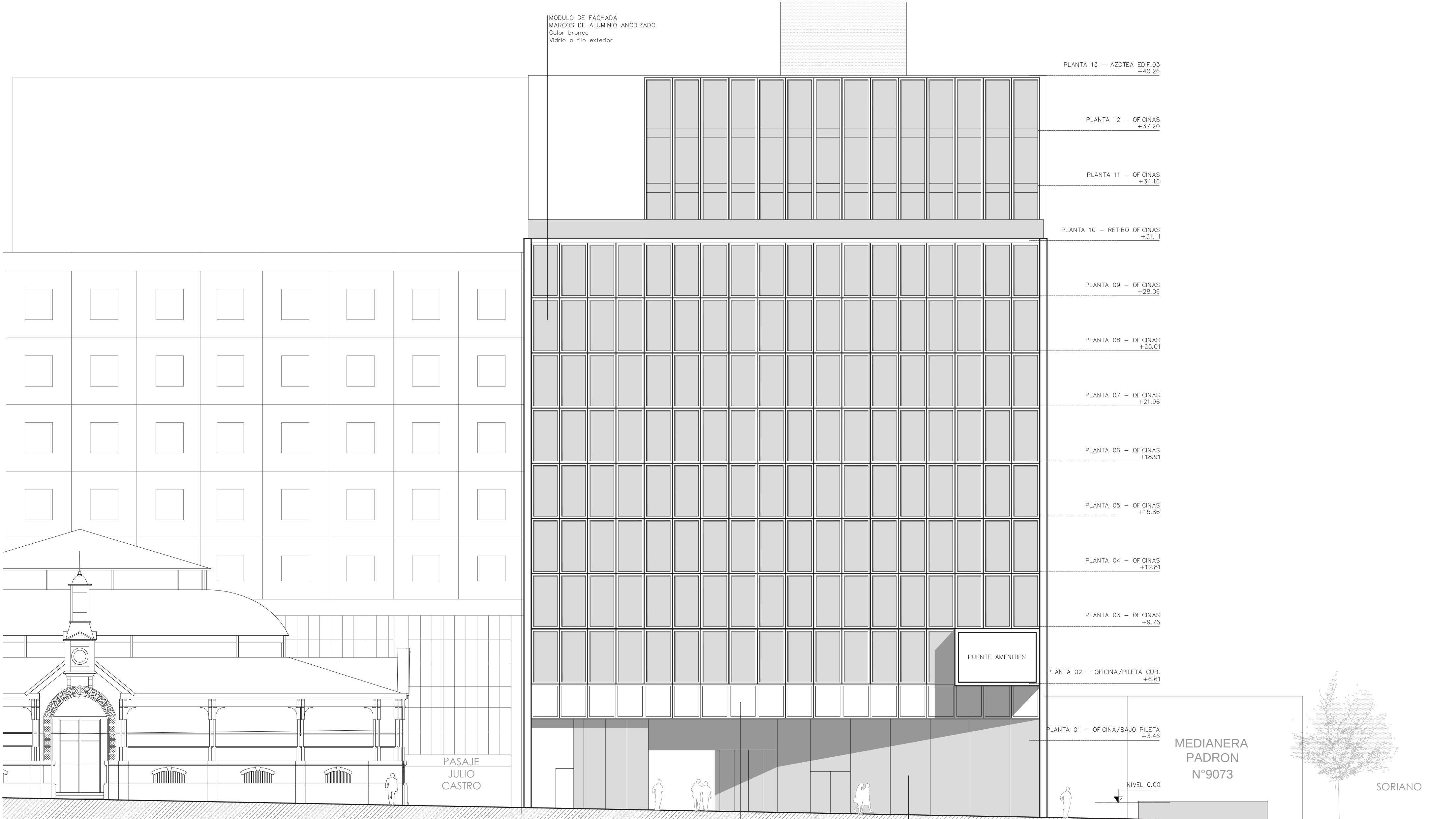
Vista Oeste Edificio 3
