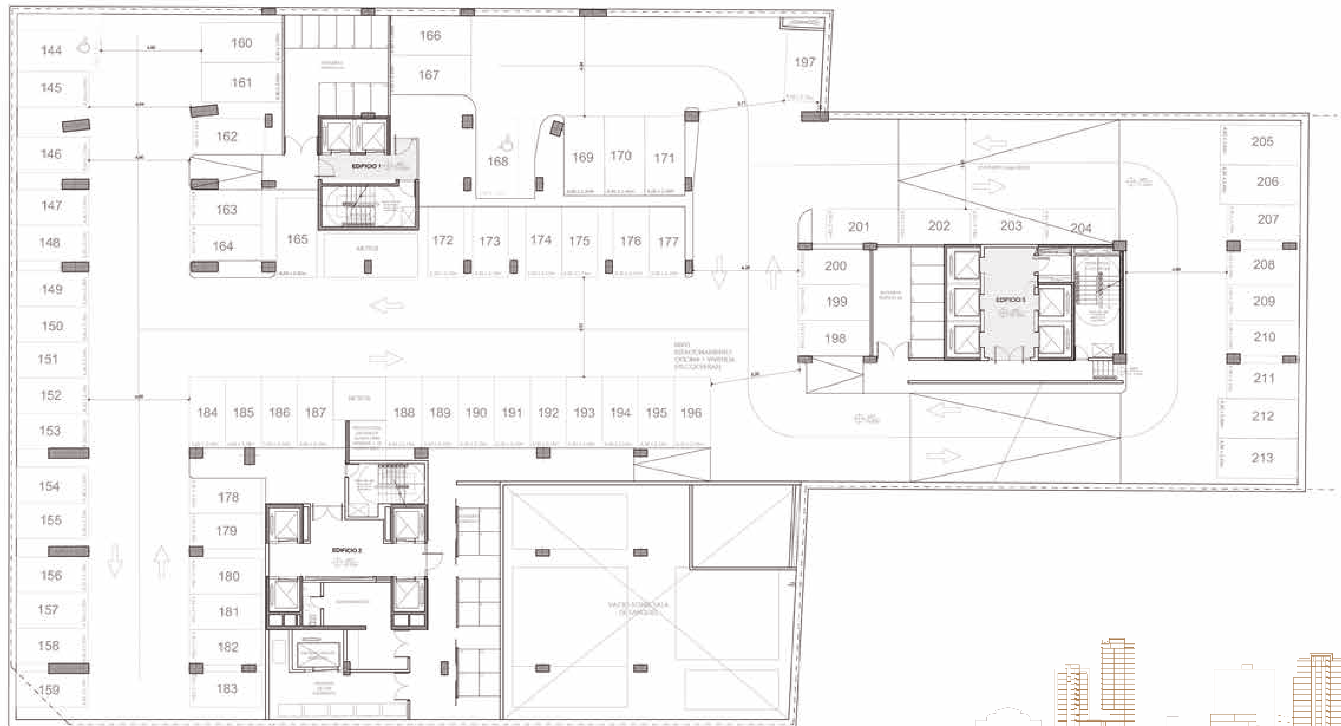
Planta Nivel -3
