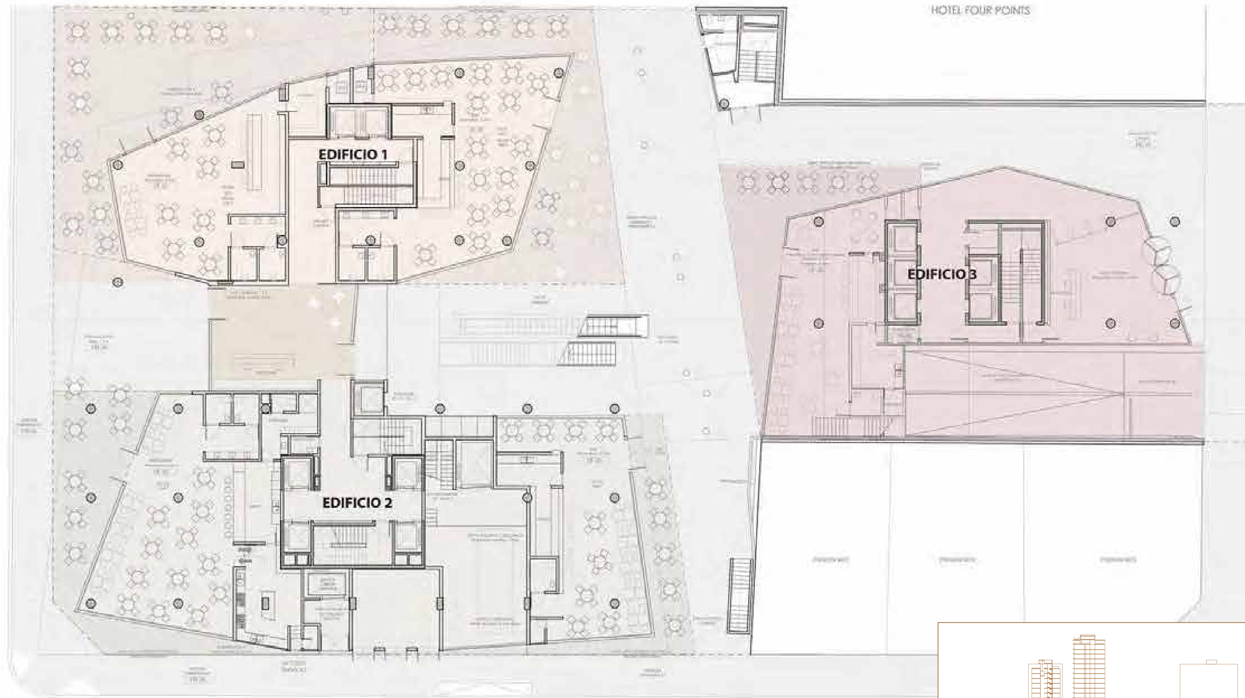
Planta Nivel PB / Accesos
