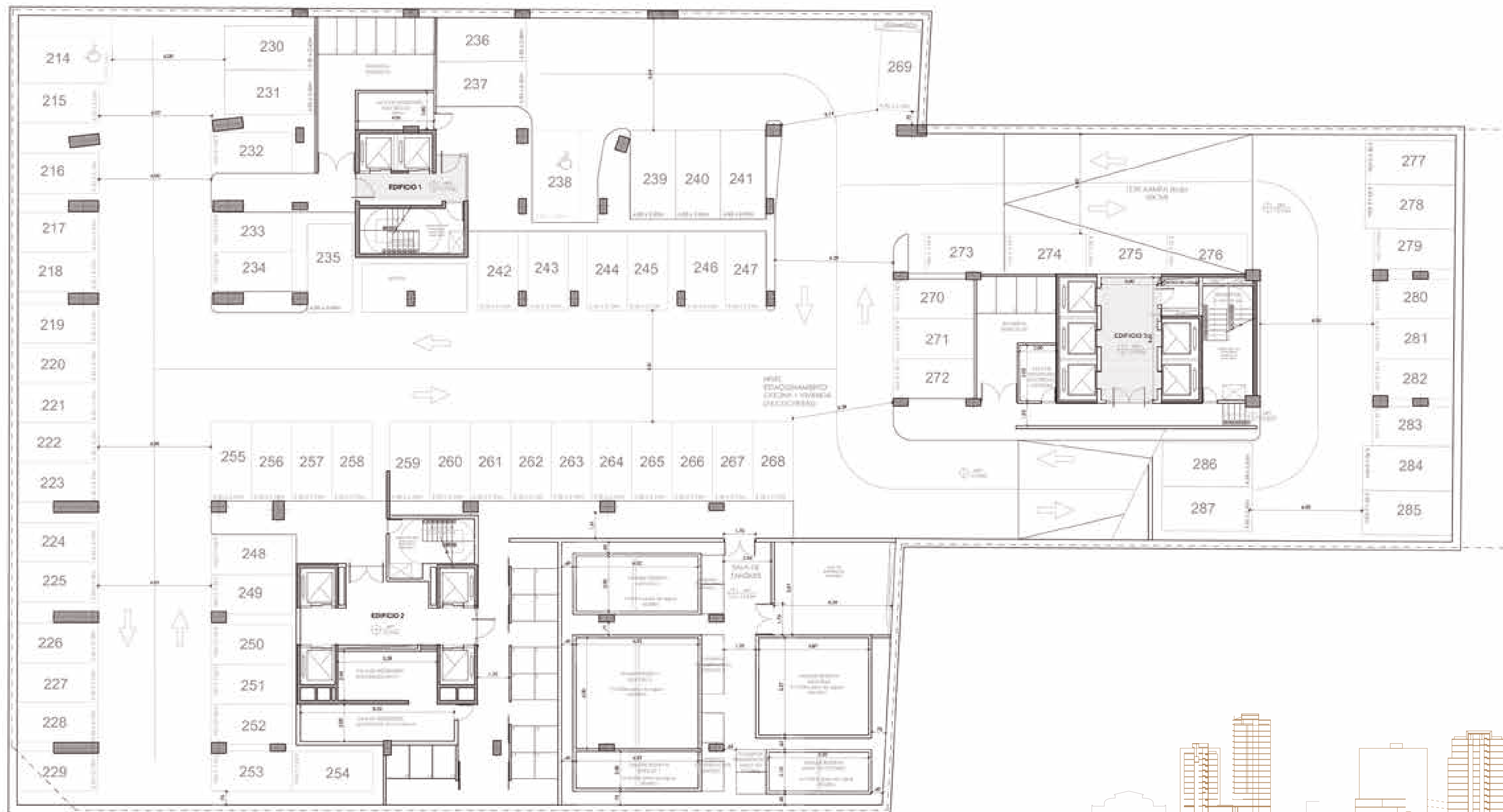
Planta Nivel -4
